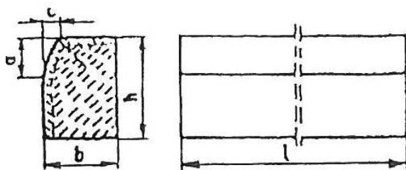
Tablica 1. Wymiary krawężników betonowych
